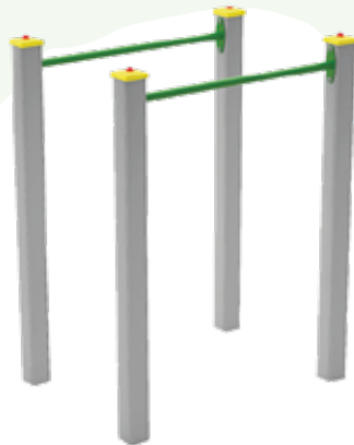
Parallele in alluminio Ingombro: 109x79x142h cm
