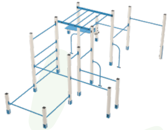
Workout Ingombro: 325x162x241h cm 488x323x241h cm 640x625x241h cm
