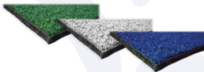
Erba sintetica multicolore Altezza: 22-27-32-37-42 mm Larghezza del rotolo: 3,70 - 4,10 mt
